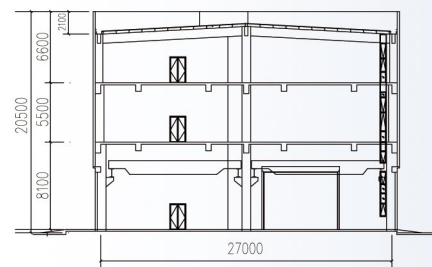
7#/10#/12#厂房剖面图
