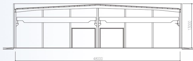
9#厂房剖面图
