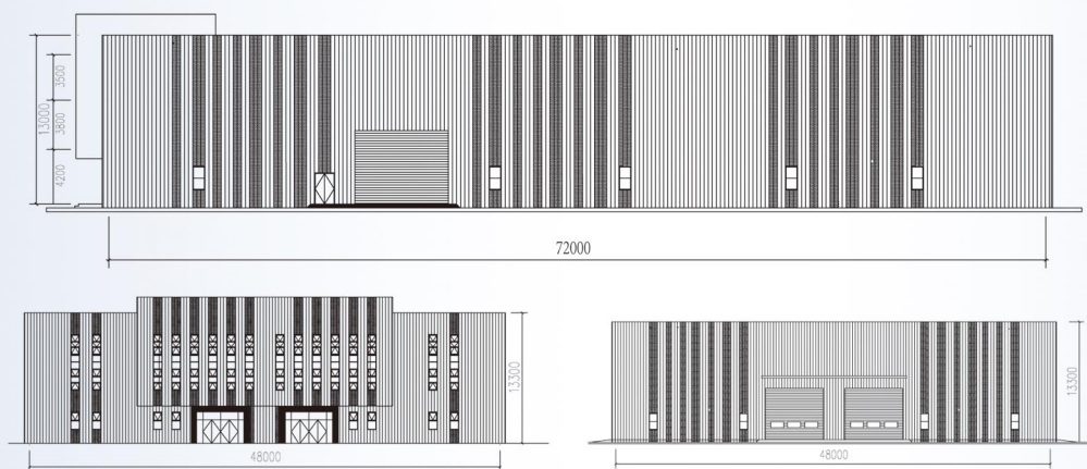
8#厂房立面图
