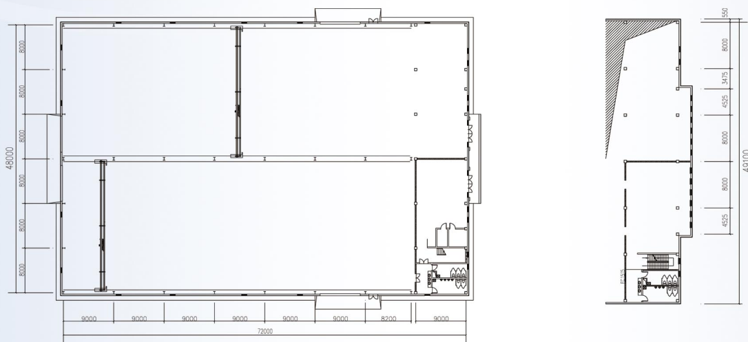
8#厂房平面图
