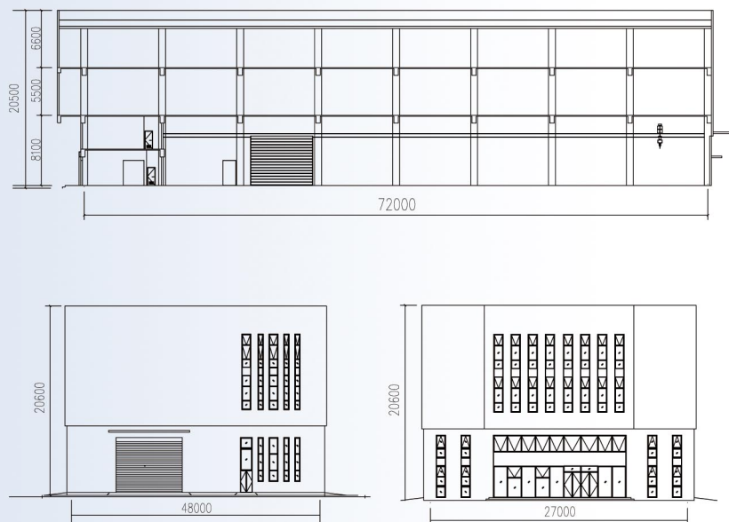
7#/10#/12#厂房立面图
