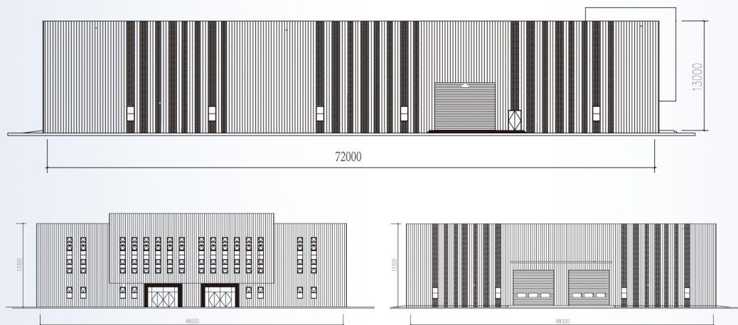
9#厂房立面图
