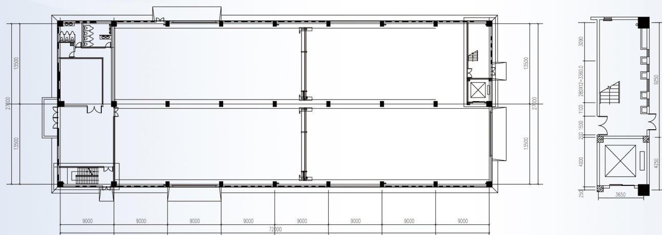
7#/10#/12#厂房平面图
