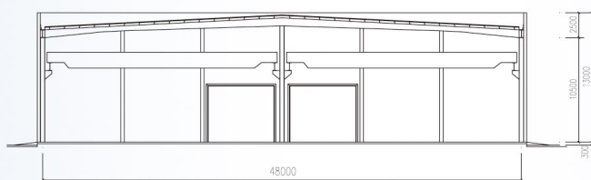
8#厂房剖面图
