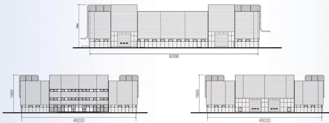
5#/6#/7#/8#厂房（C型）立面图
