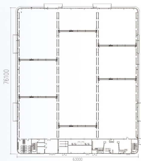
11#厂房（E型）平面图
