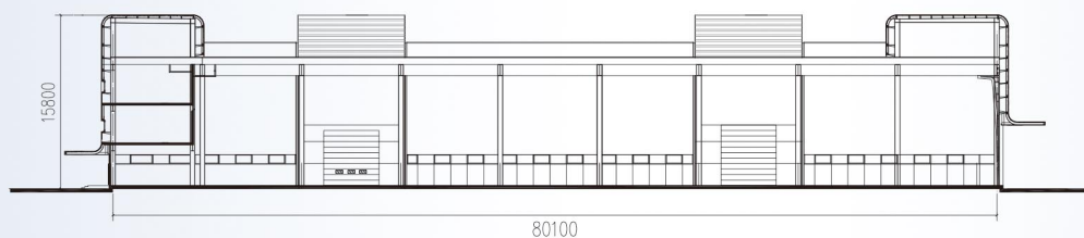
3#/4#厂房（B型）剖面图
