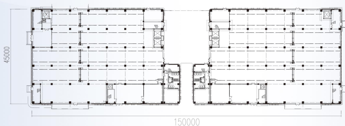
12#厂房（F型）平面图
