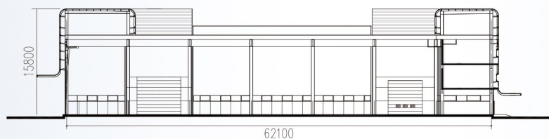
5#/6#/7#/8#厂房（C型）剖面图
