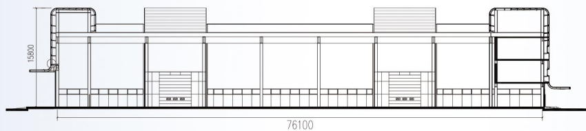
11#厂房（E型）剖面图
