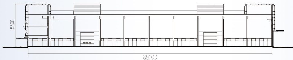
1#/2#厂房（A型）剖面图
