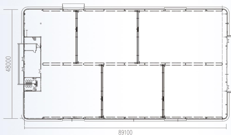
1#/2#厂房（A型）平面图
