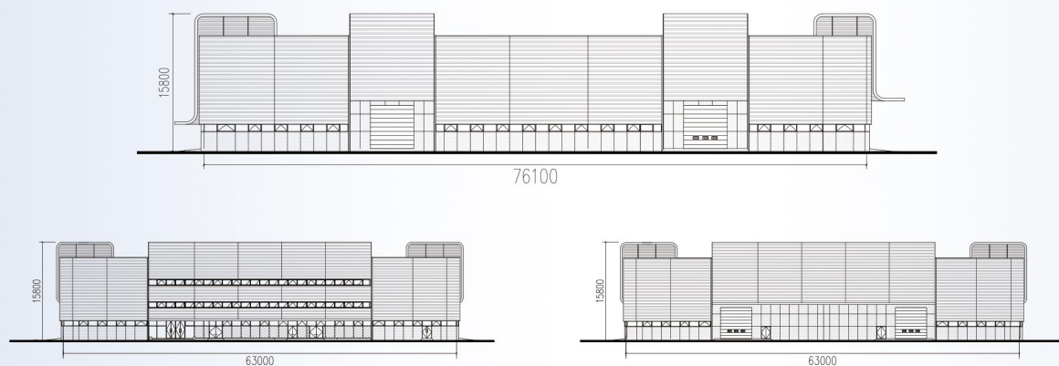
11#厂房（E型）立面图
