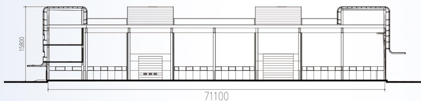
9#/10#厂房（D型）剖面图
